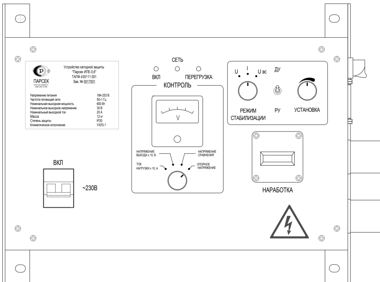
Рисунок 1 – Внешний вид устройства «Парсек ИПЕ-0,6»
